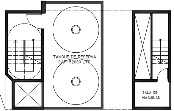
PLANTA TANQUES
